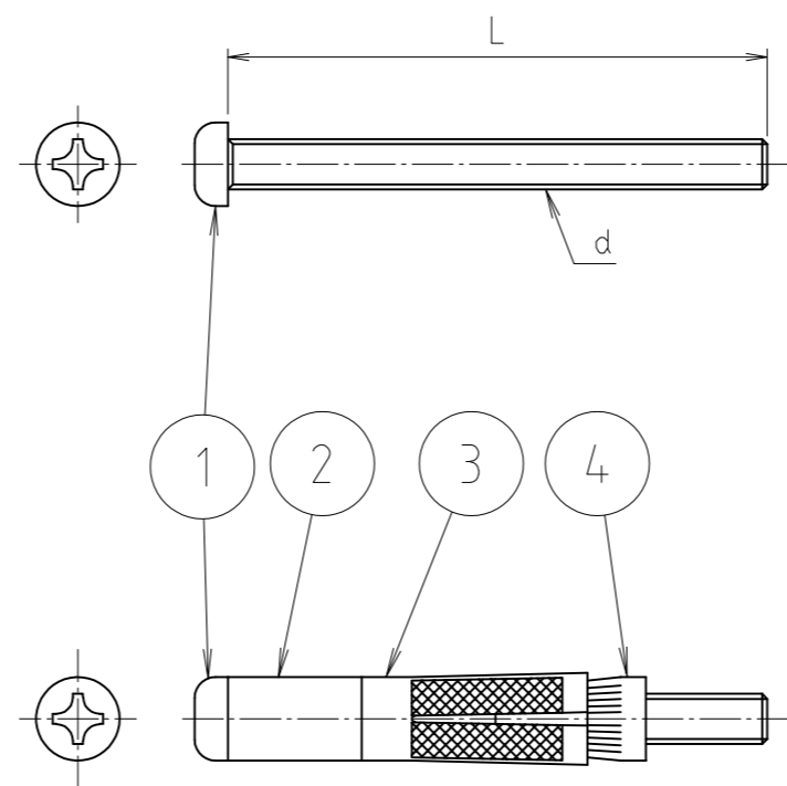
■組立図
