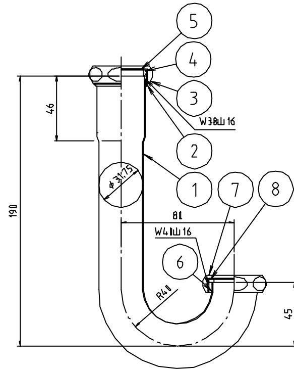
寸法：32×80×190
